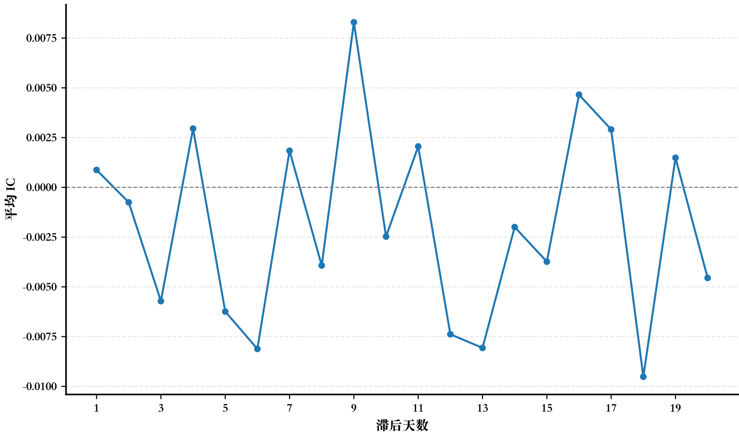
IC 衰减: amihud_illiq_z
