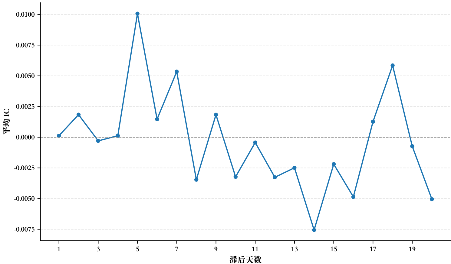
IC 衰减: max_ret_1m_z
