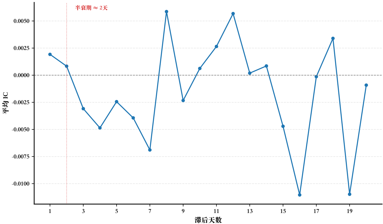
IC 衰减: momentum_12m_z
