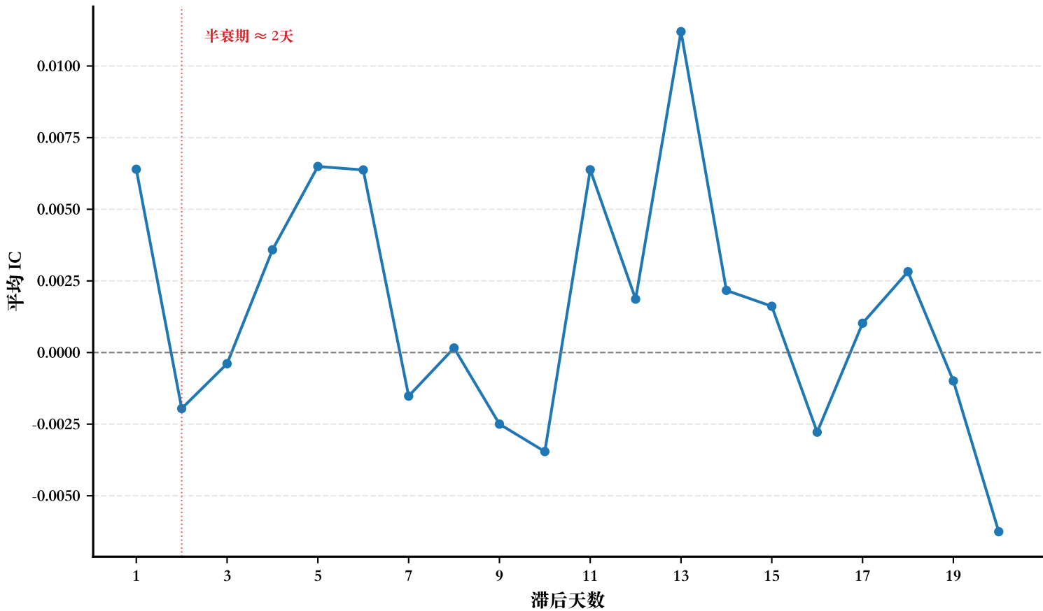
IC 衰减: st_reversal_1w_z
