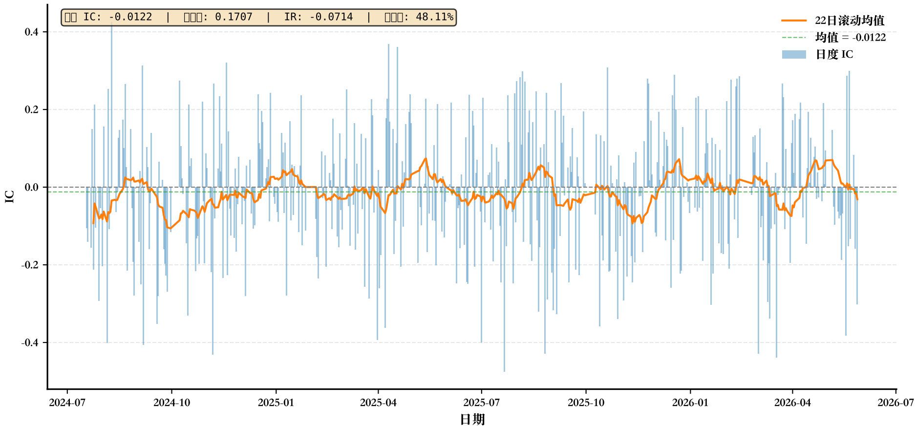
IC 时序: momentum_12m_z
