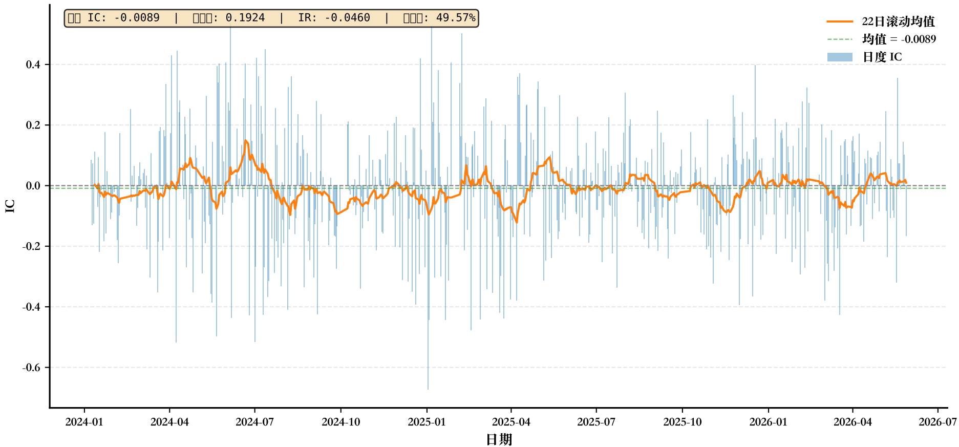
IC 时序: momentum_6m_z
