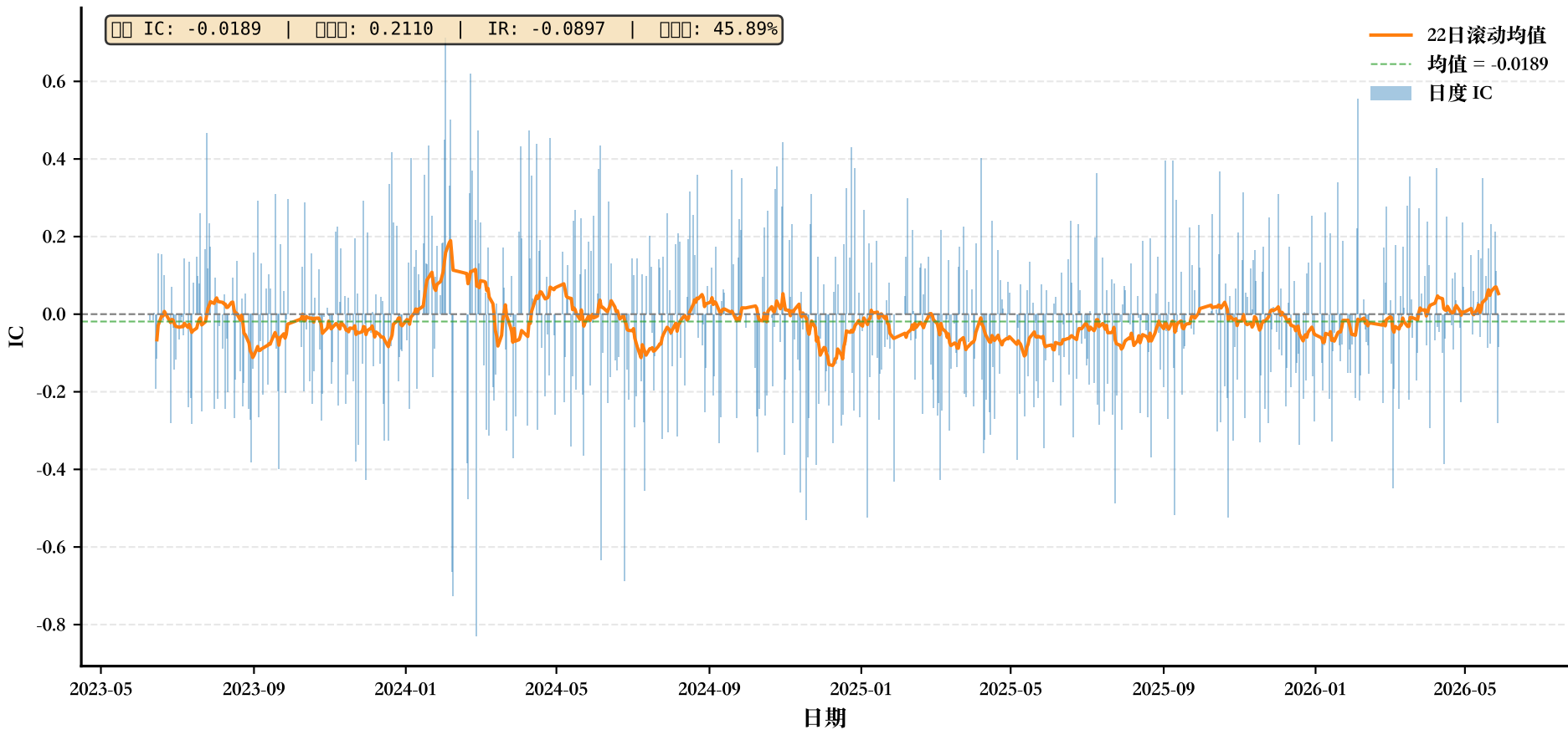
IC 时序: st_reversal_1w_z
