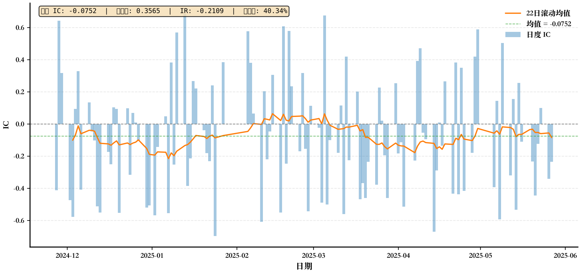
IC 时序: ivol_capm_z
