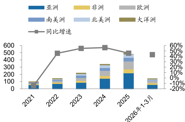
图 10：2021-2026Q1 变压器出口金额（亿元）及同比增速
