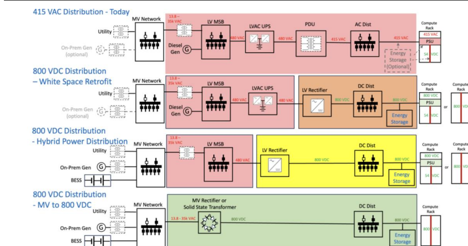
图 21：英伟达800V直流白皮书中展示的数据中心架构演进规划图
