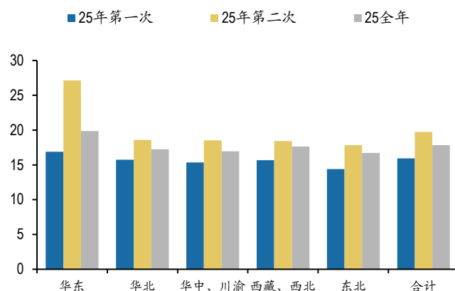
图 18: 25年第二批次融合环网箱联采均价已有所回升 (单位: 万元/套)
