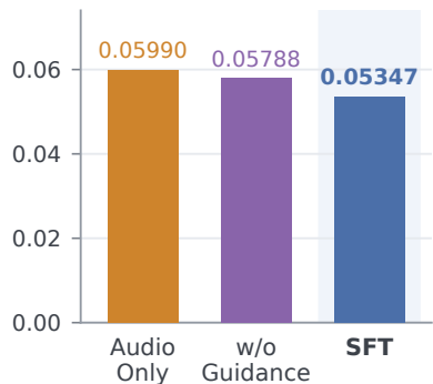
(b) MAE ↓
