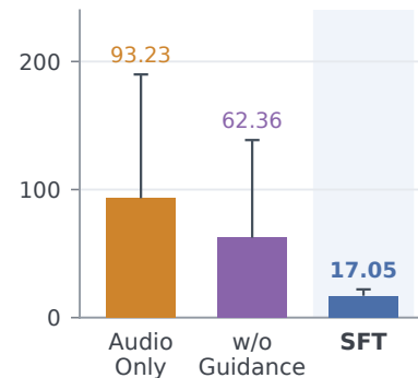
(d) WInD ↓
