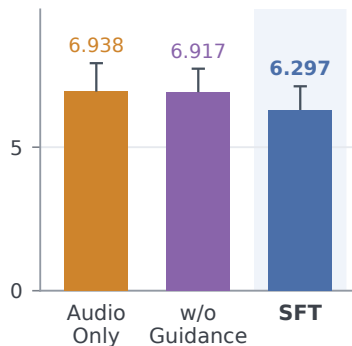
(e) LMD ↓
