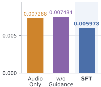
(a) MSE ↓
