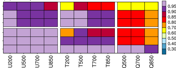
(d) Temporal correlation, mid-latitudes
