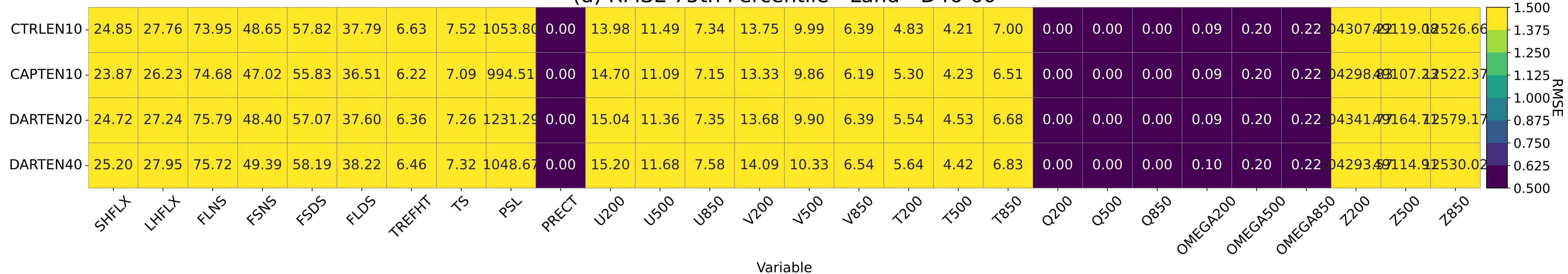
(d) RMSE 75th Percentile - Land - D46-60
