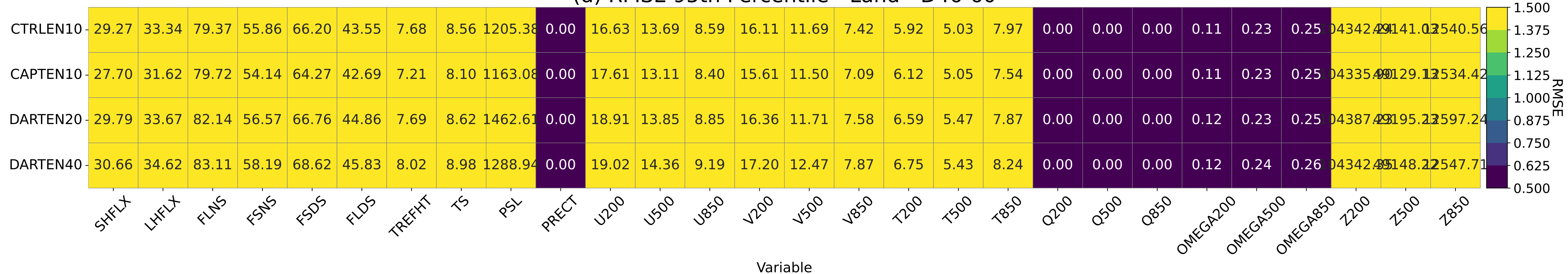
(d) RMSE 95th Percentile - Land - D46-60
