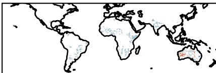
ERA5-ESACCI | D16-30
