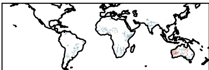
ERA5-ESACCI | D16-30
