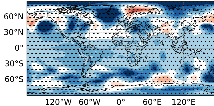
EAM-DART (ENS=20)
