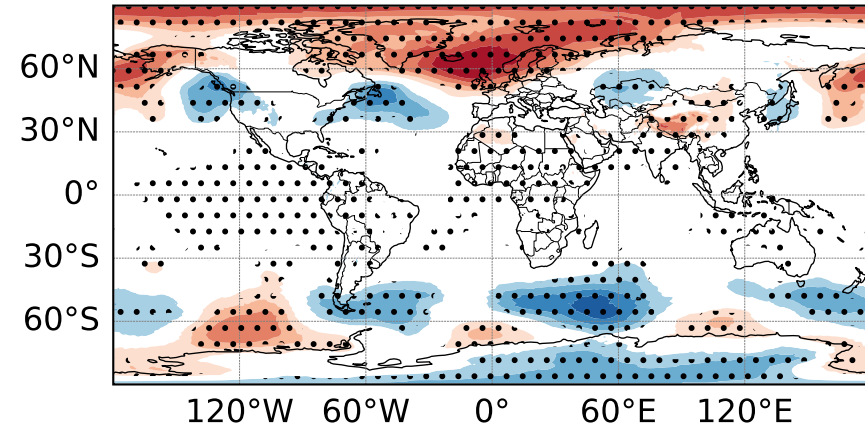
CTRL (ENS=10)
