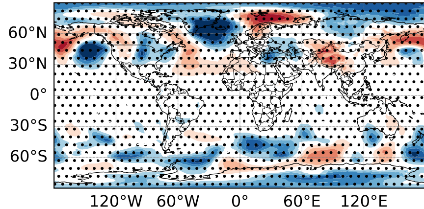
EAM-DART (ENS=40)
