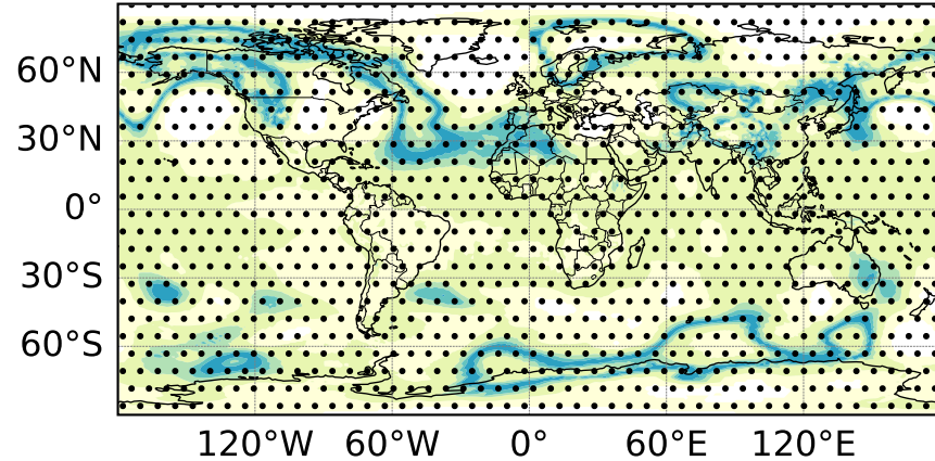
EAM-DART (ENS=20)
