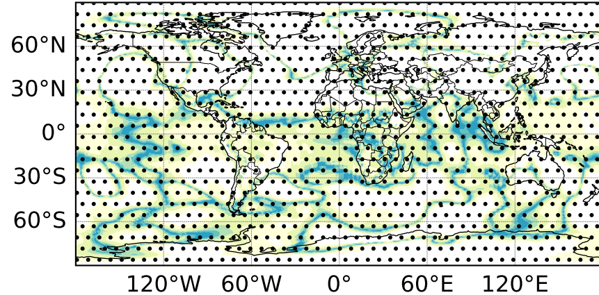
EAM-DART (ENS=40)
