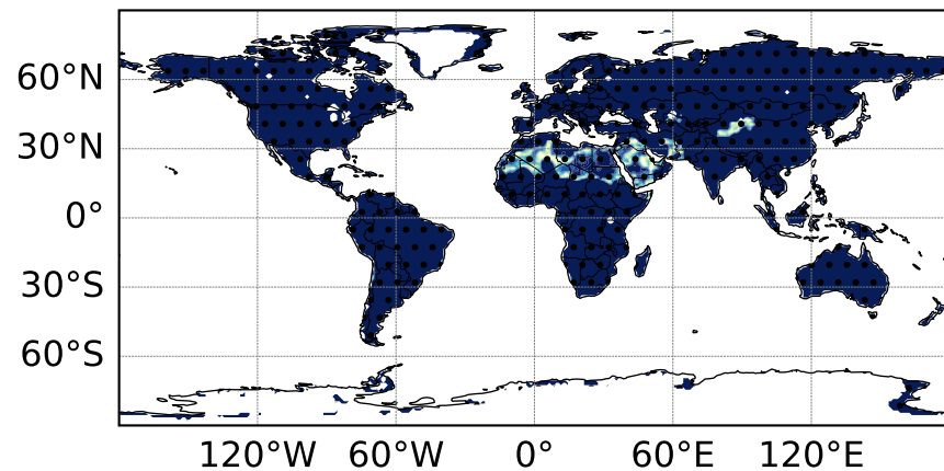
EAM-DART (ENS=20)
