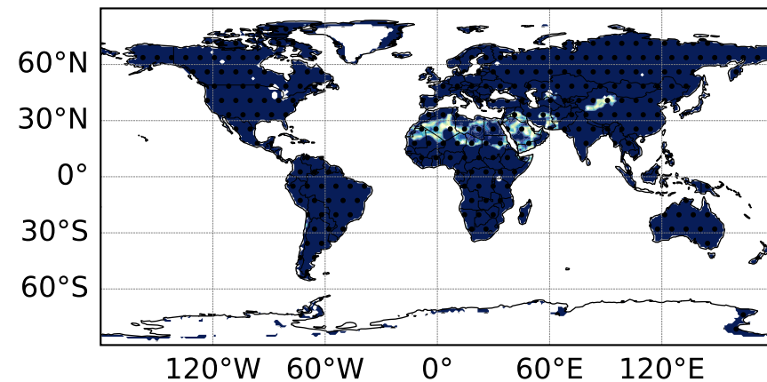
CTRL (ENS=10)
