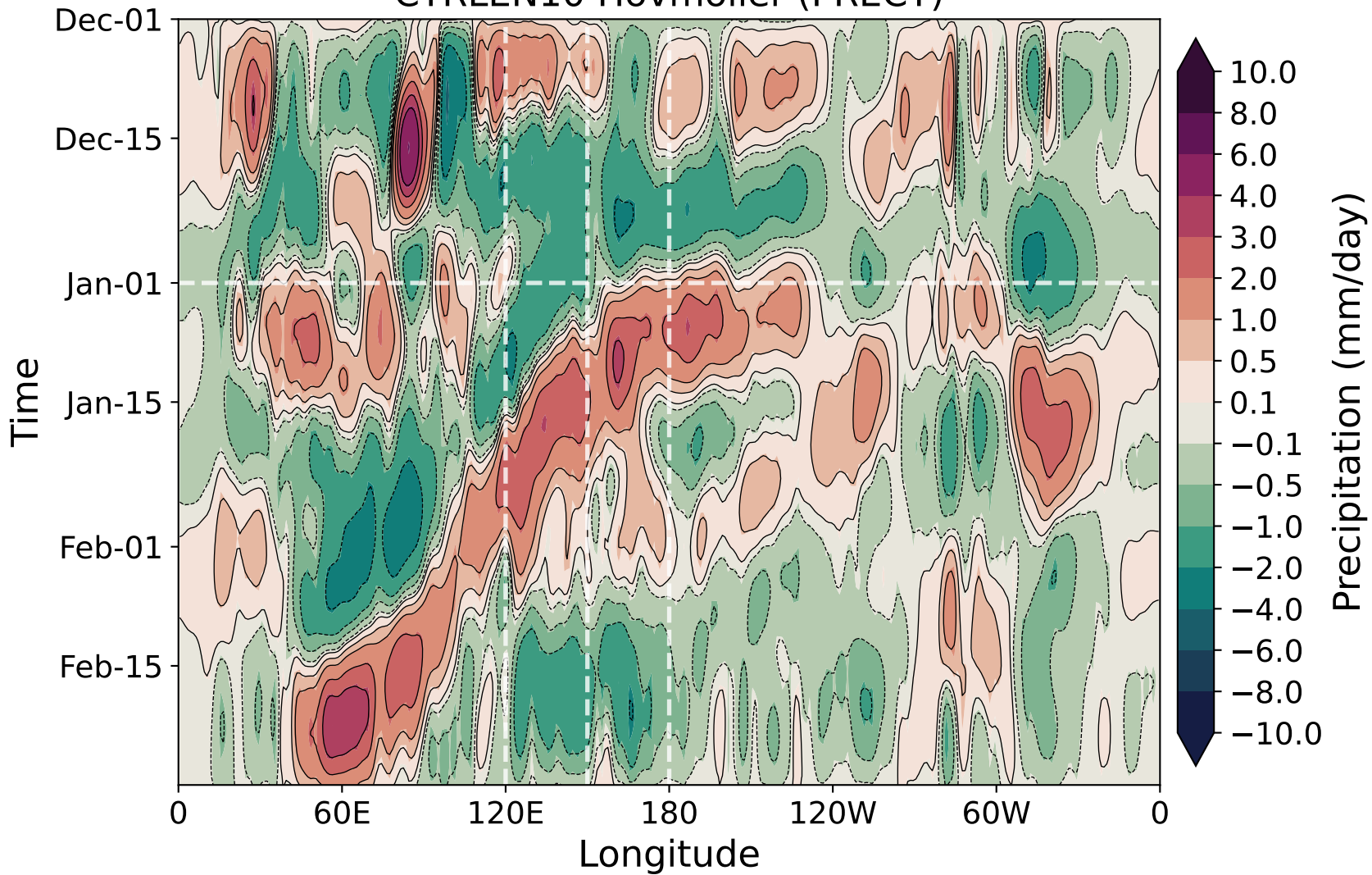
CTRLLEN10 Hovmoller (PRECT)
