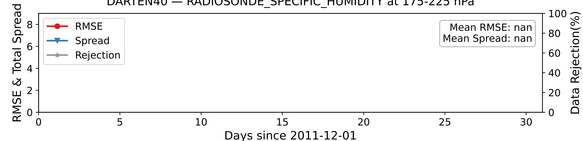
DARTEN40 — RADIOSONDE_SPECIFIC_HUMIDITY at 175-225 hPa
