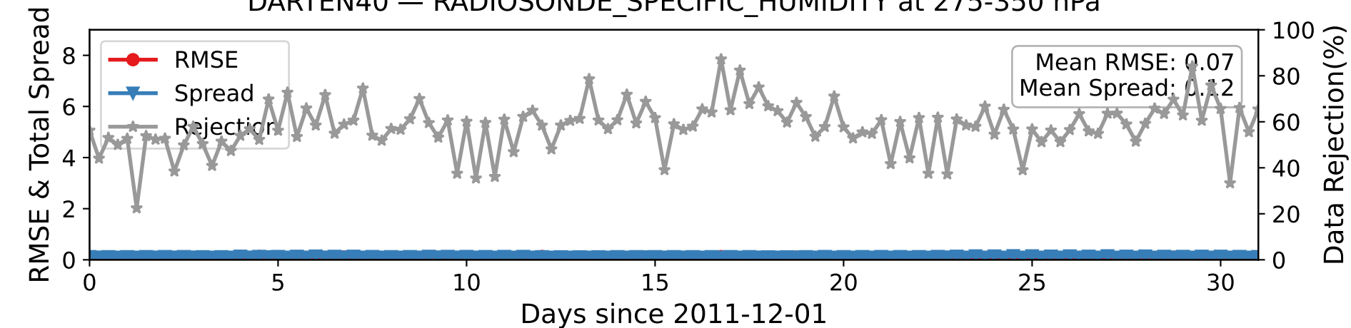
DARTEN40 — RADIOSONDE_SPECIFIC_HUMIDITY at 275-350 hPa
