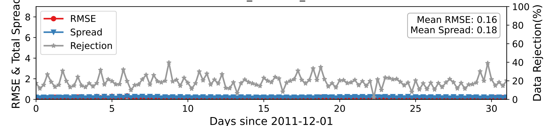
DARTEN40 — RADIOSONDE_SPECIFIC_HUMIDITY at 350-450 hPa
