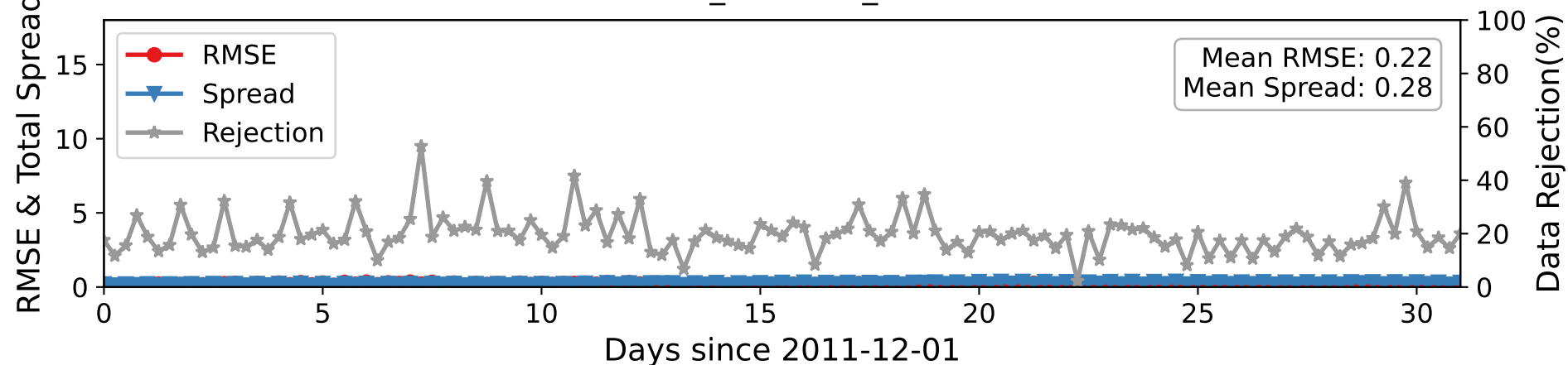
DARTEN10 — RADIOSONDE_SPECIFIC_HUMIDITY at 350-450 hPa
