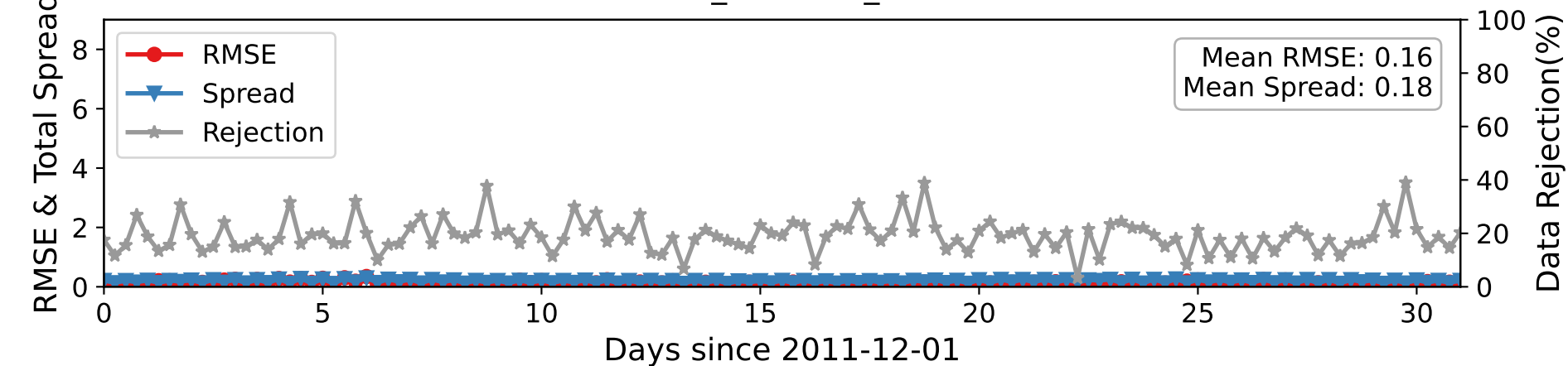
DARTEN40 — RADIOSONDE_SPECIFIC_HUMIDITY at 350-450 hPa
