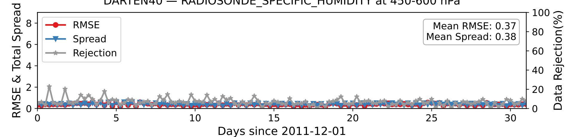
DARTEN40 — RADIOSONDE_SPECIFIC_HUMIDITY at 450-600 hPa
