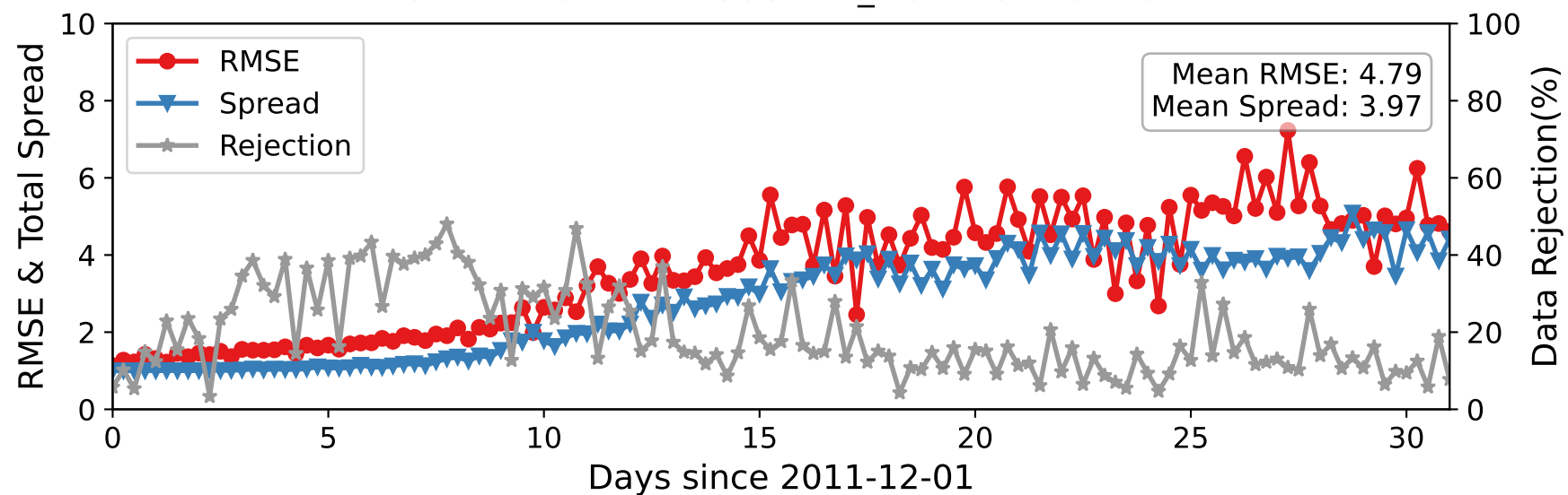
CTRLLEN10 — RADIOSONDE_T at 125-175 hPa
