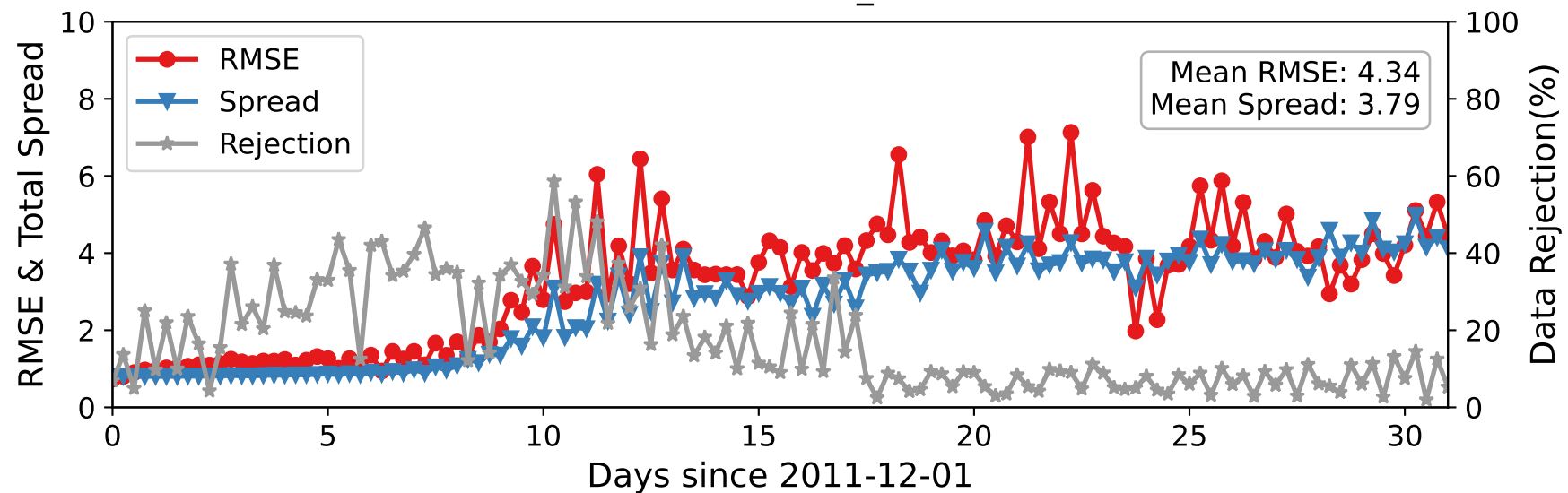
CTRLLEN10 — RADIOSONDE_T at 450-600 hPa
