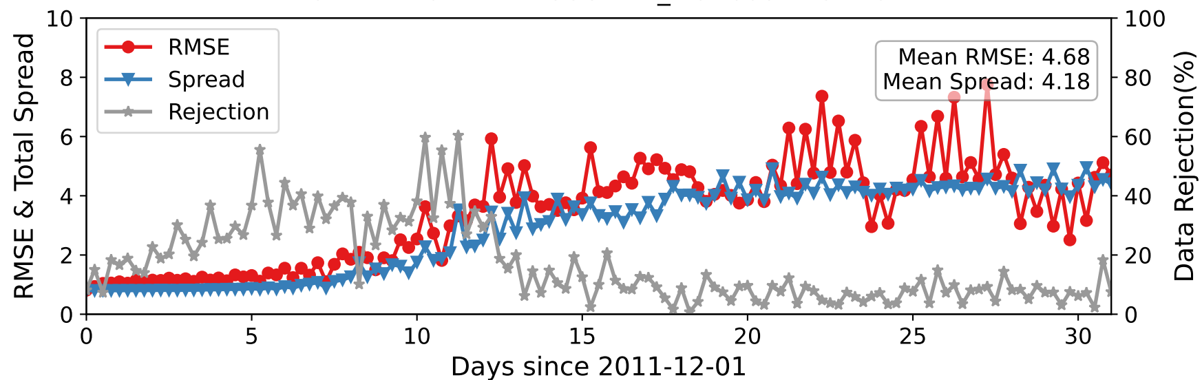
CTRLLEN10 — RADIOSONDE_T at 600-775 hPa
