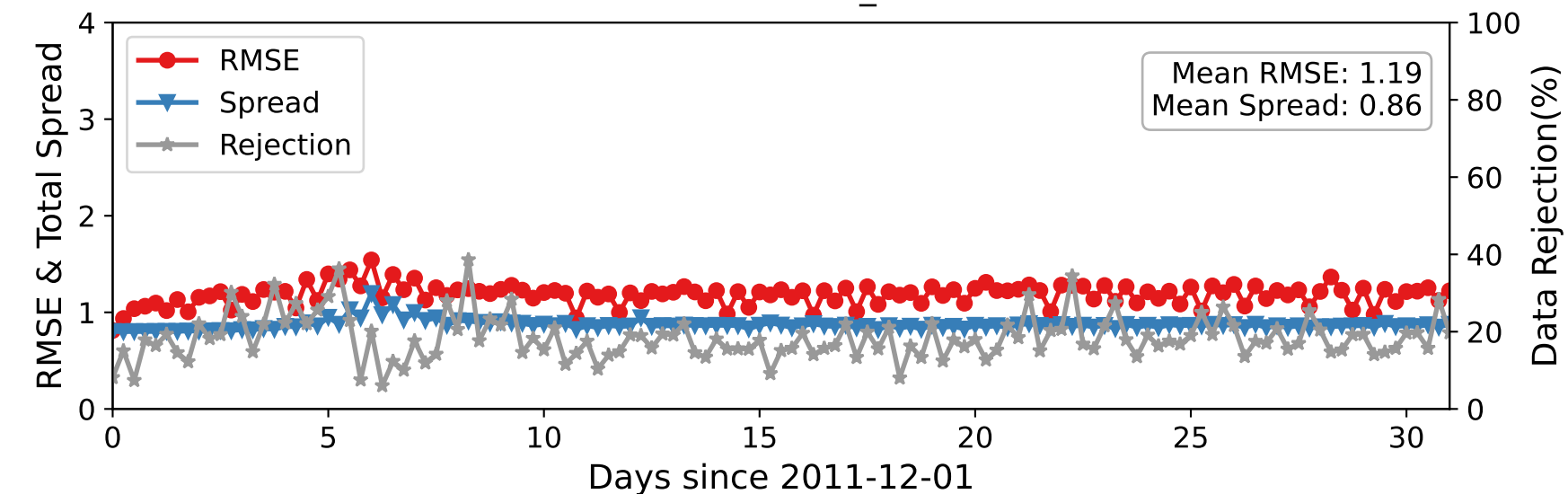
DARTEN40 — RADIOSONDE_T at 600-775 hPa
