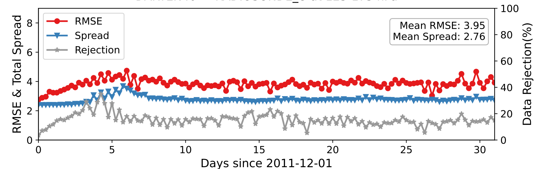
DARTEN40 — RADIOSONDE_U at 125-175 hPa
