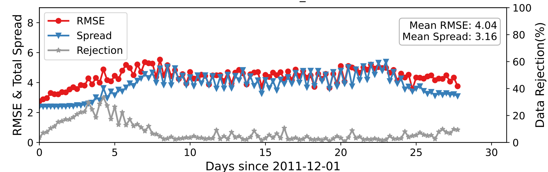
DARTEN10 — RADIOSONDE_U at 125-175 hPa
