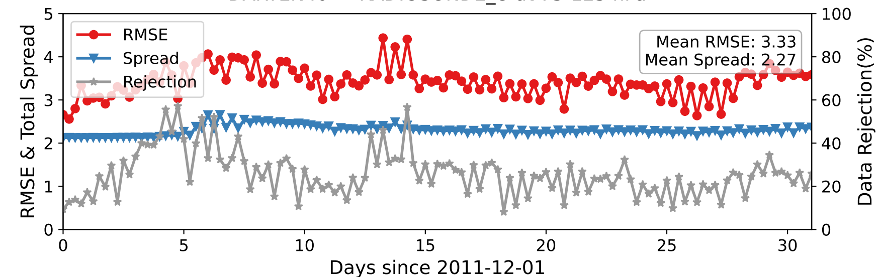
DARTEN40 — RADIOSONDE_U at 75-125 hPa
