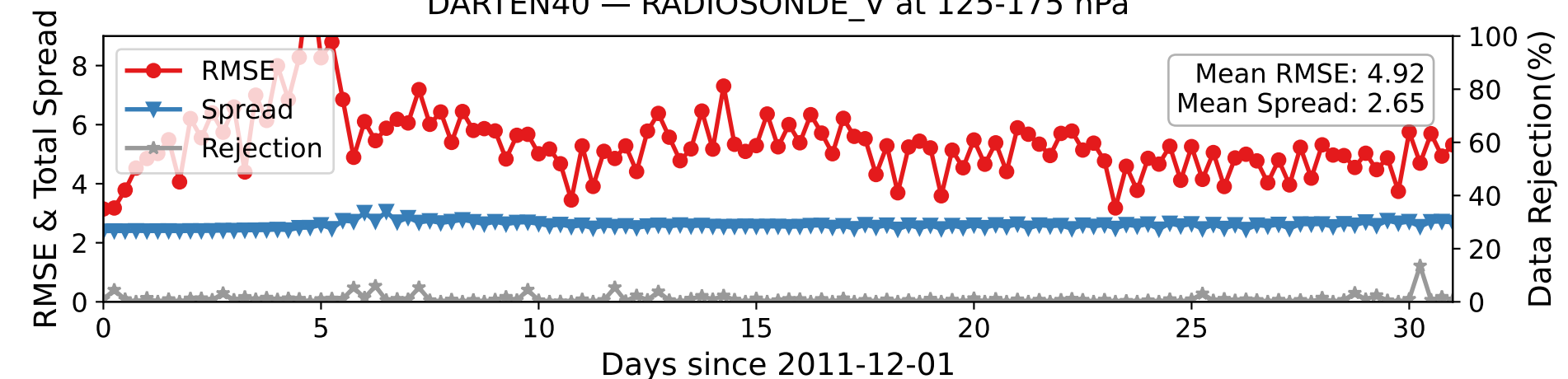
DARTEN40 — RADIOSONDE_V at 125-175 hPa
