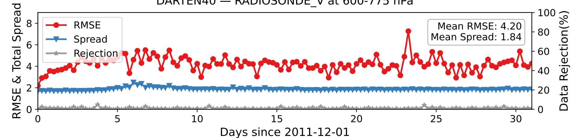
DARTEN40 — RADIOSONDE_V at 600-775 hPa
