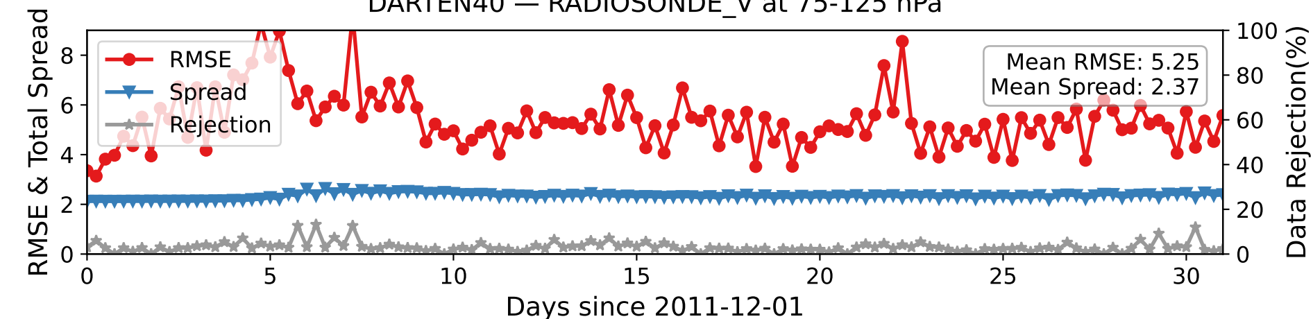
DARTEN40 — RADIOSONDE_V at 75-125 hPa
