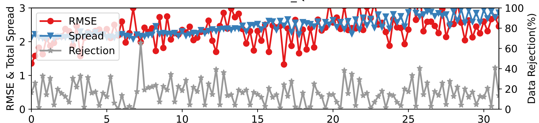
CTRLEN10 — RADIOSONDE_Q at 600-775 hPa
