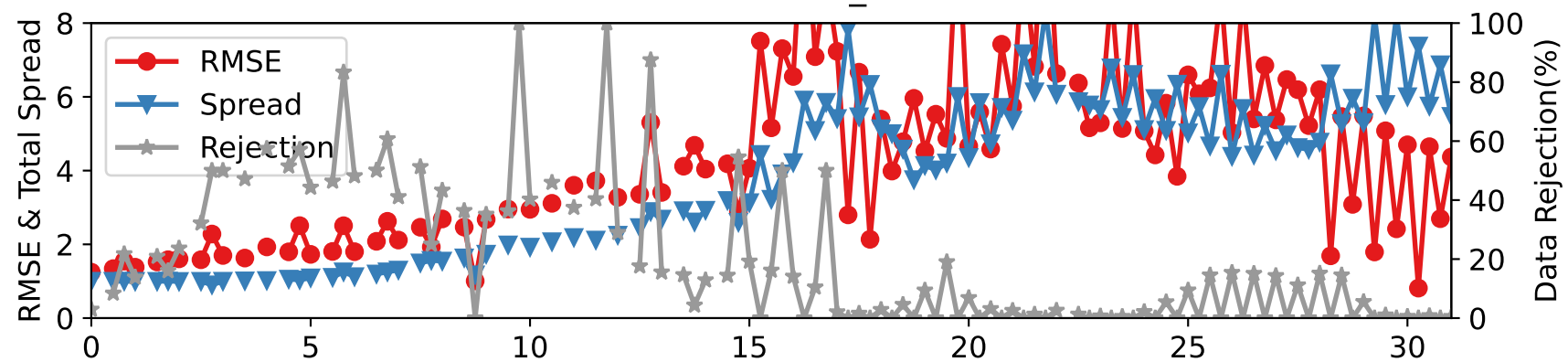
CTRLLEN10 — RADIOSONDE_T at 125-175 hPa
