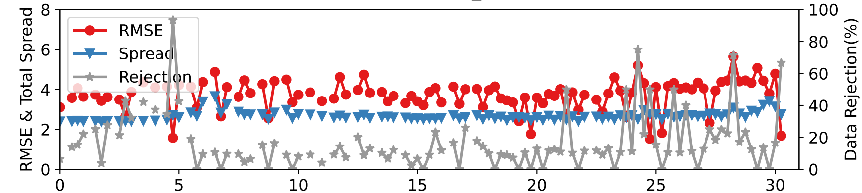
DARTEN40 — RADIOSONDE_V at 125-175 hPa
