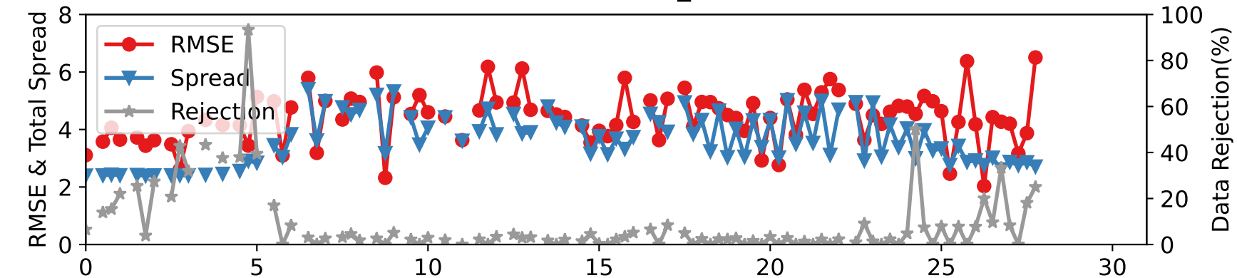
DARTEN10 — RADIOSONDE_V at 125-175 hPa
