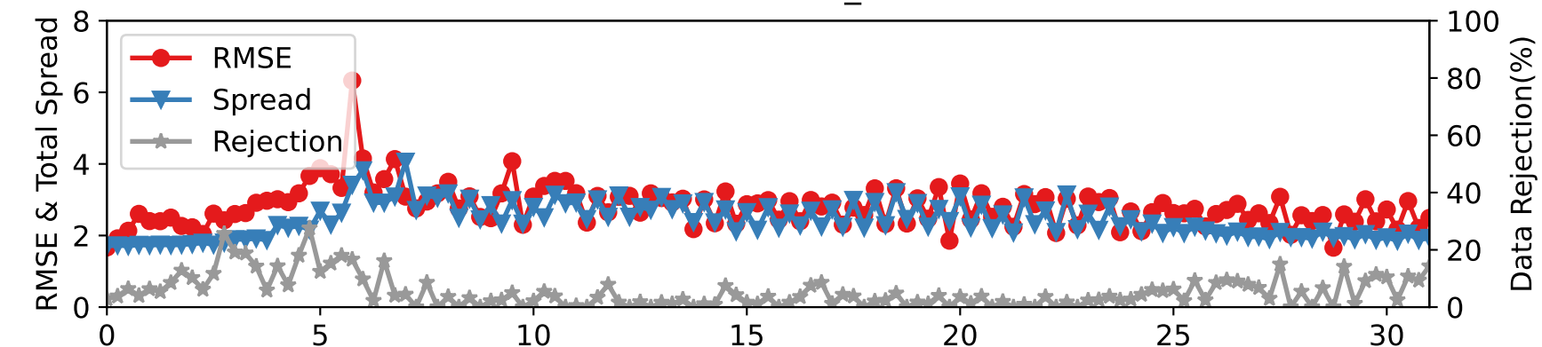
DARTEN20 — RADIOSONDE_V at 600-775 hPa
