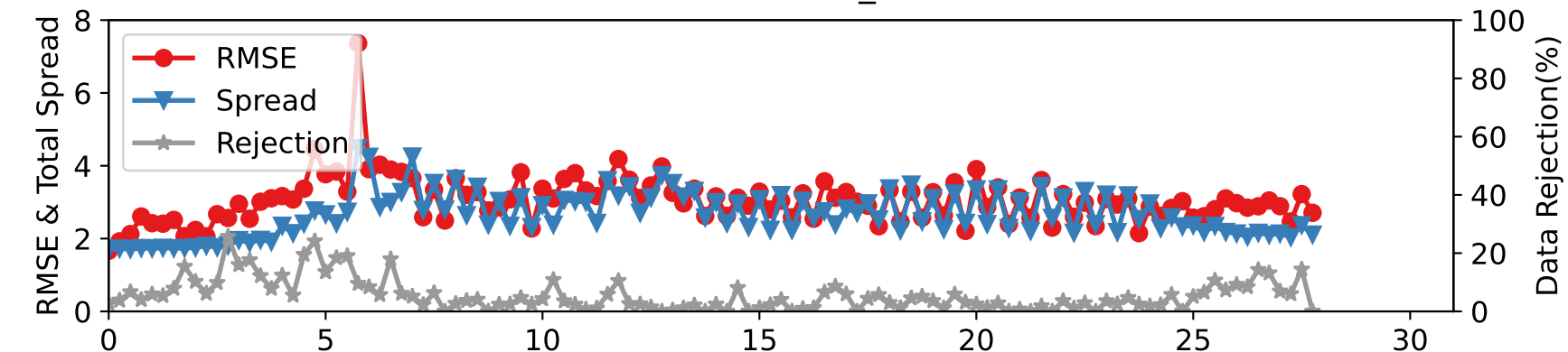
DARTEN10 — RADIOSONDE_V at 600-775 hPa
