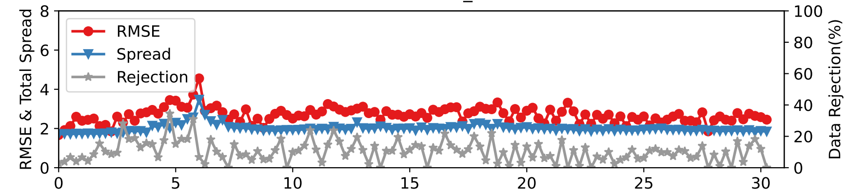
DARTEN40 — RADIOSONDE_V at 600-775 hPa
