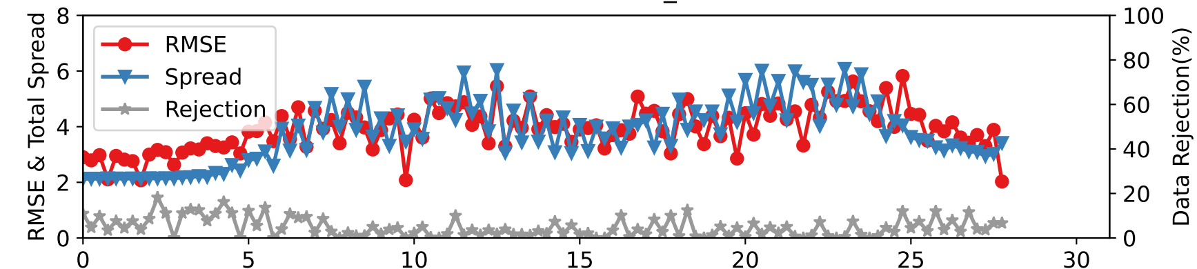
DARTEN10 — RADIOSONDE_V at 75-125 hPa
