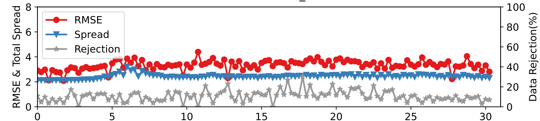
DARTEN40 — RADIOSONDE_V at 75-125 hPa
