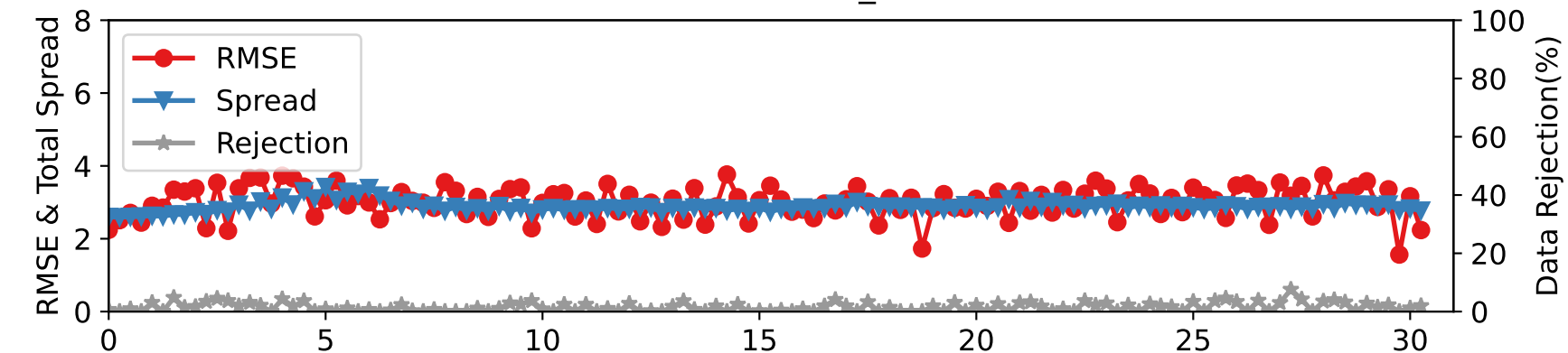
DARTEN40 — RADIOSONDE_V at 350-450 hPa
