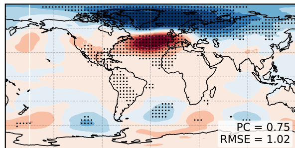
(d) NARRM_r0125 NAO (DJF,1985-2014)
