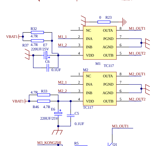
功放部分
