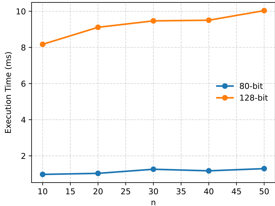
(d) Time Cost of GroupKeyUpdate
