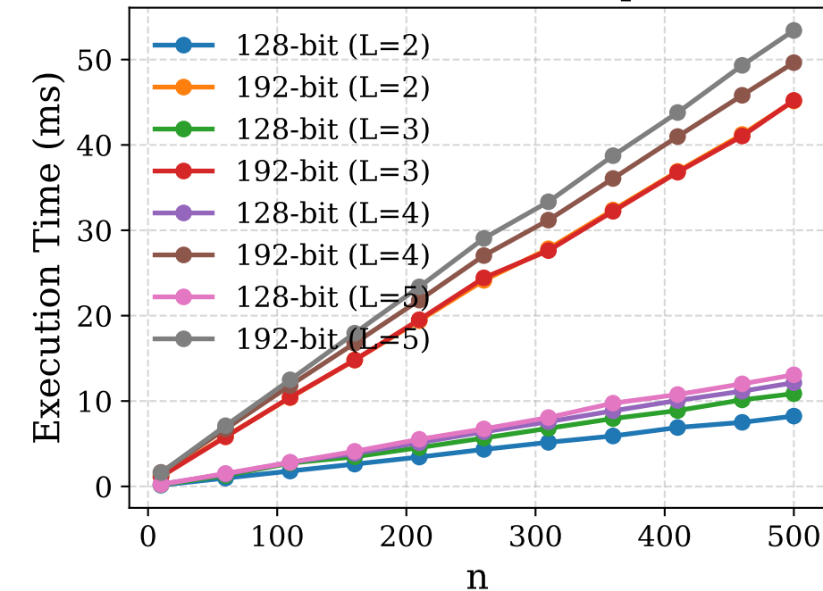
(d) Time Cost of Split
