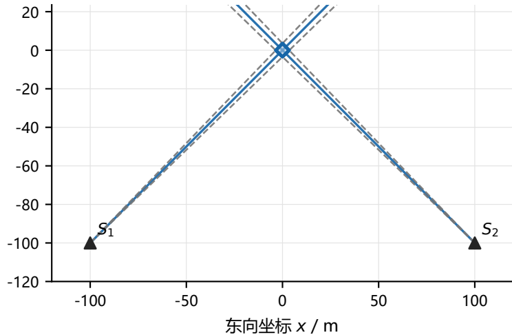
(a) 全局测向交会几何（边界采样 96 点）
