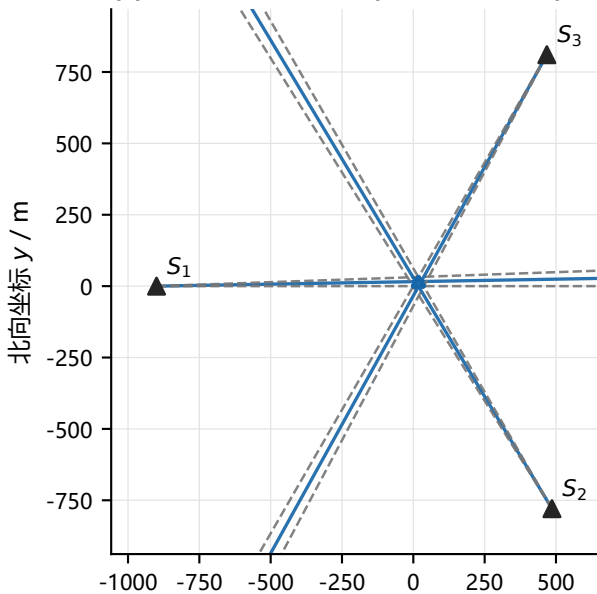
(a) 全局测向交会几何 (边界采样 72 点)
