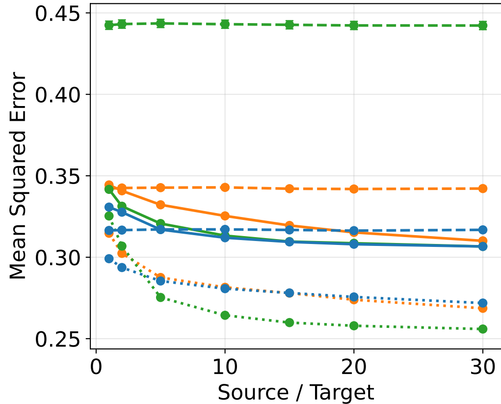
n_0 = 50
