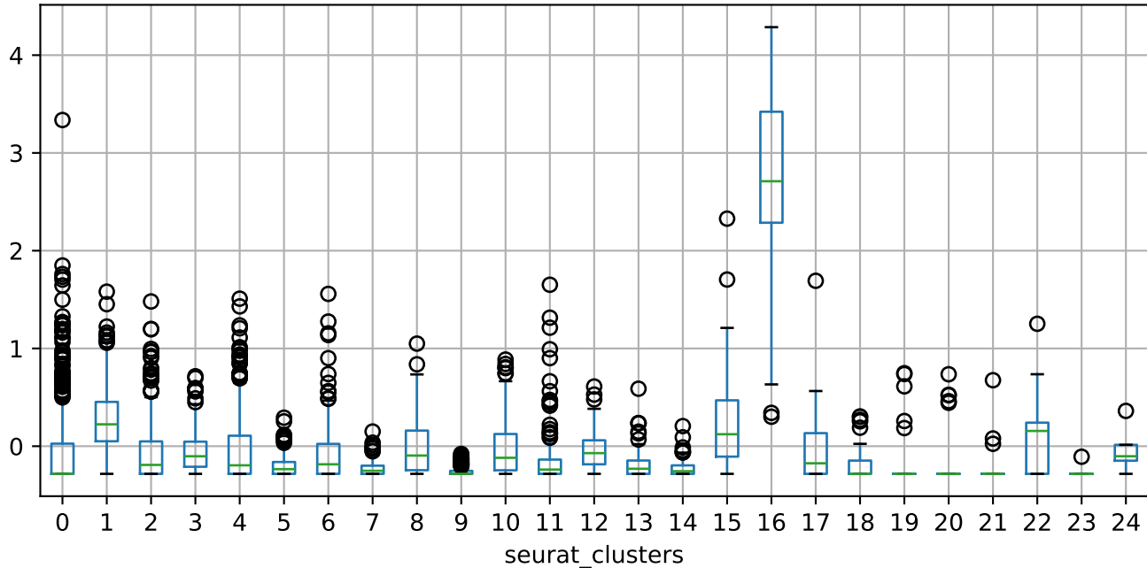
NormalScore
