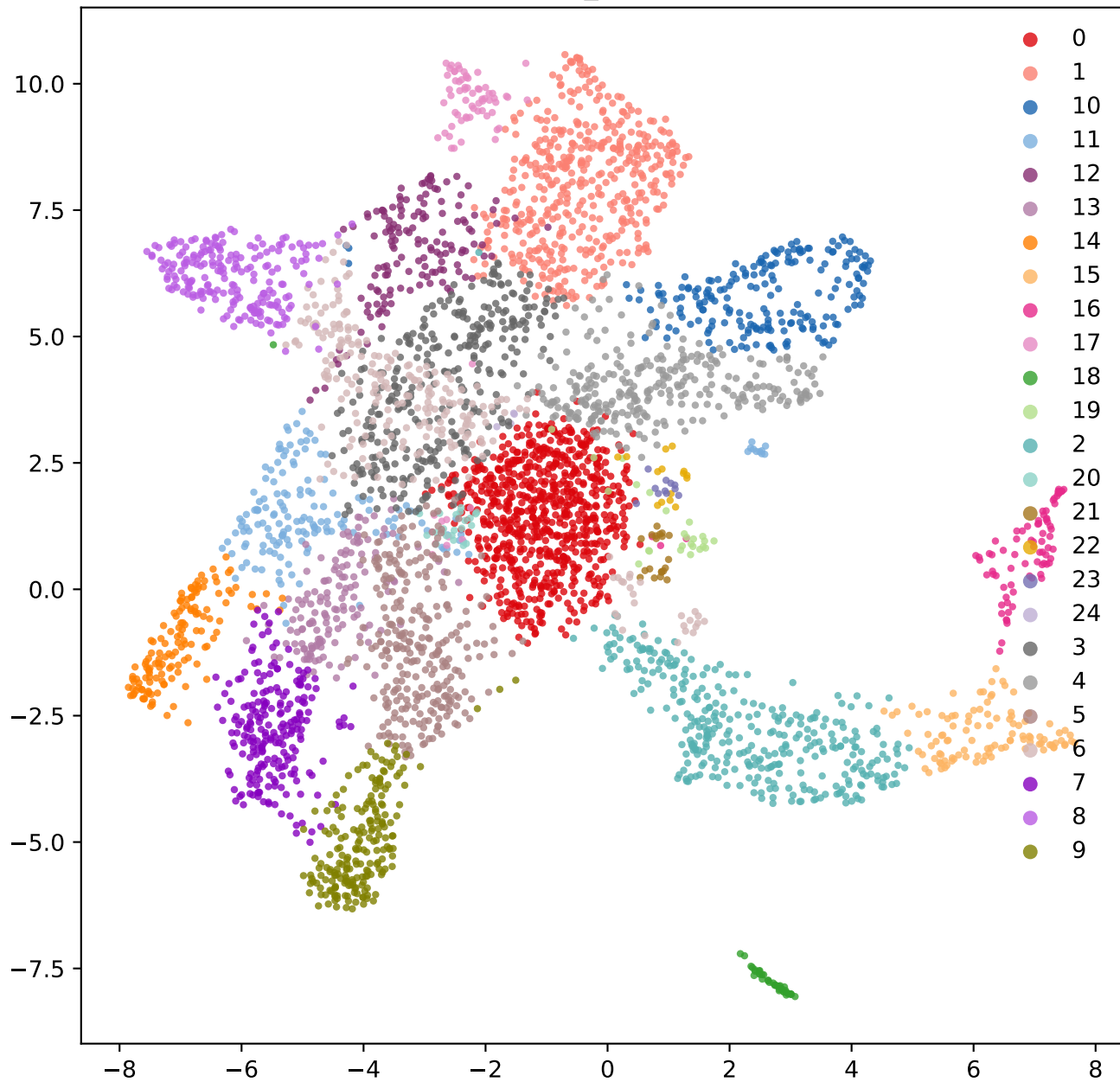
seurat_clusters
