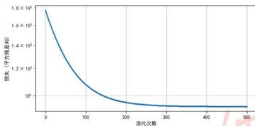
图 7: 高斯-牛顿迭代误差收敛情况
