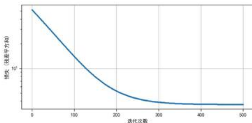
图 10: 高斯-牛顿迭代误差收敛情况
