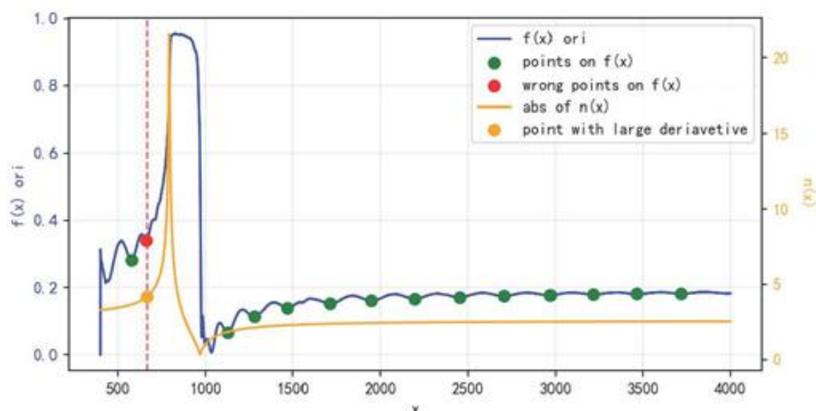
图 18: 问题 2 直接算法可疑点去除示意图
