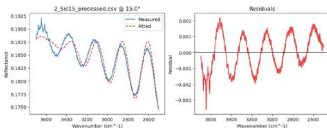
图 9 15 度-SiC 拟合结果
