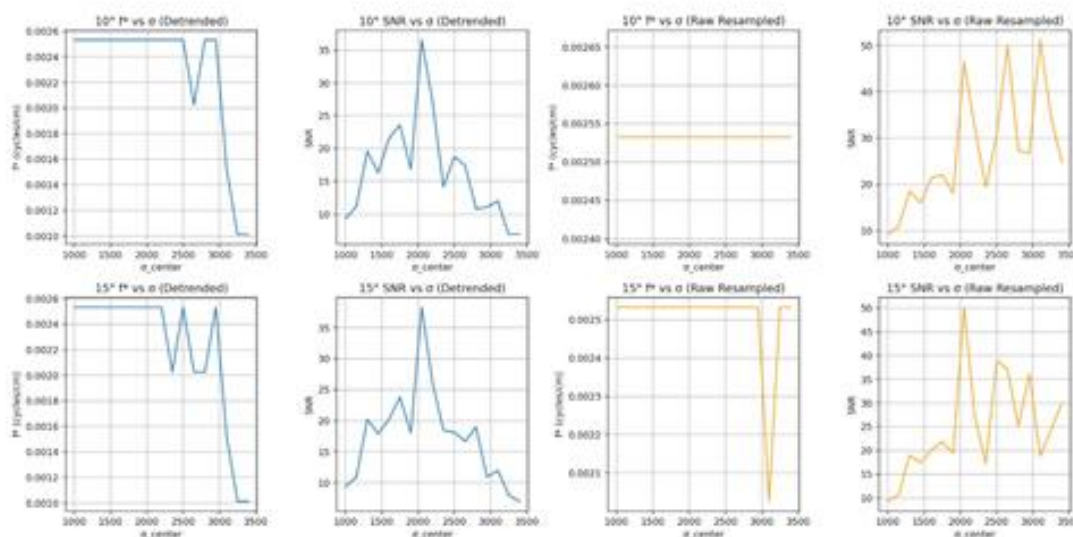
图 25 滑窗 FFT：去基线 vs. 仅重采样的 f^* 与 SNR 对比
