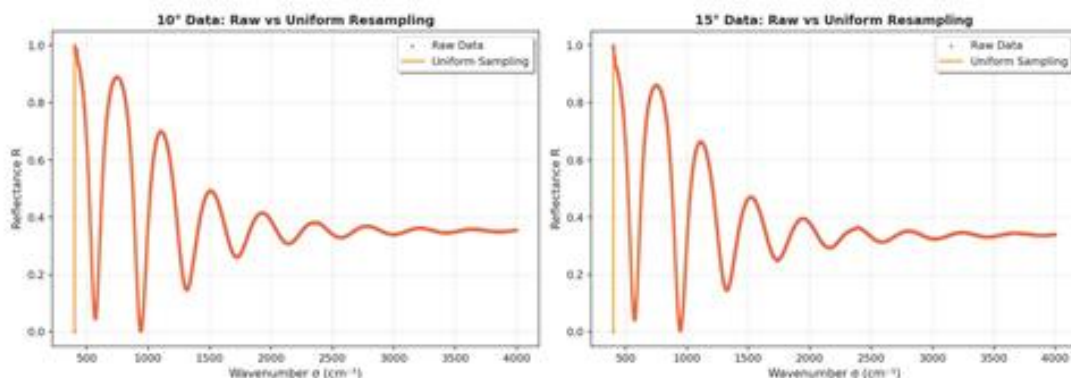
图 23 硅片反射率光谱：原始散点 vs. 等间距重采样（左：10°；右：15°）。
