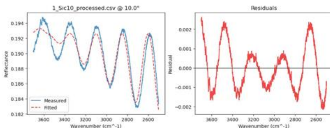
图 8 10 度-SiC 拟合结果
