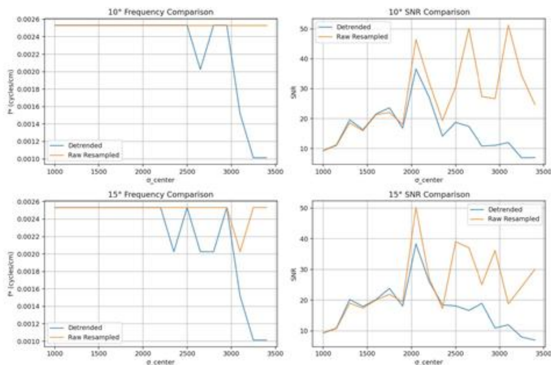
图 26 局部主频与 SNR 的叠图比较
