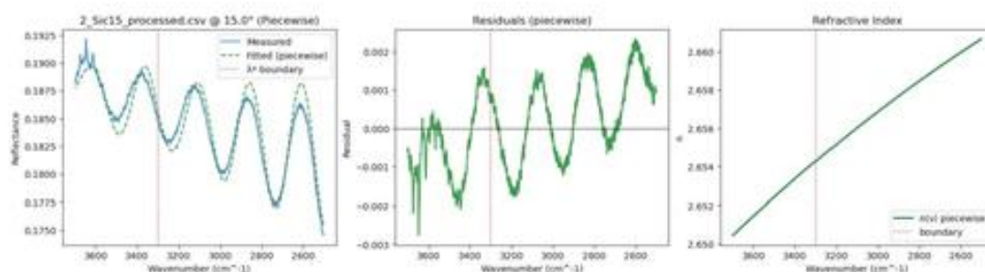
图 11 15 度-SiC 分段拟合结果
