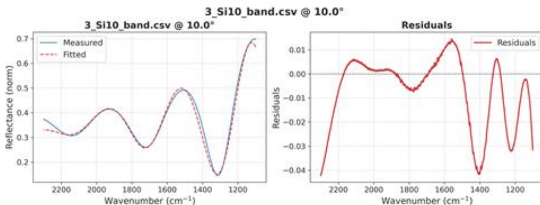
图 30 10 度-Si 拟合结果
