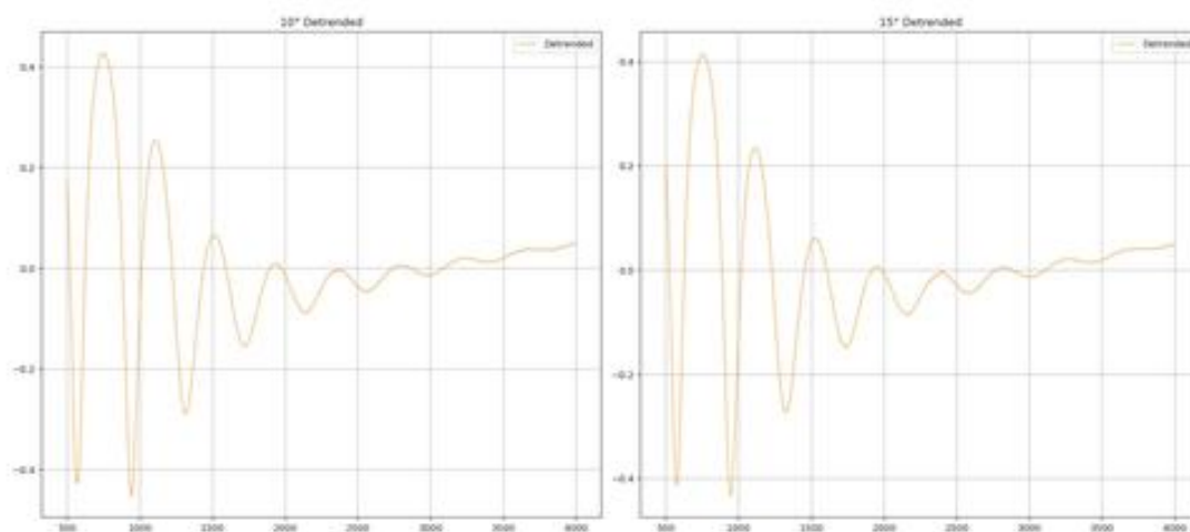
图 24 轻量去基线后的硅片反射率光谱
