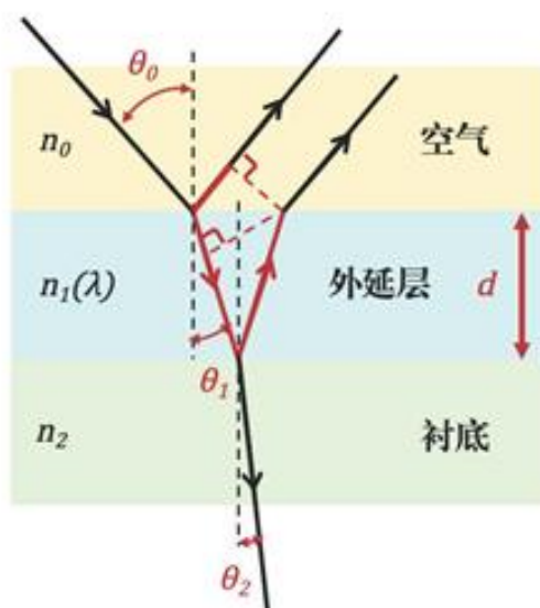
图1 两光束干涉模型的光路示意图
