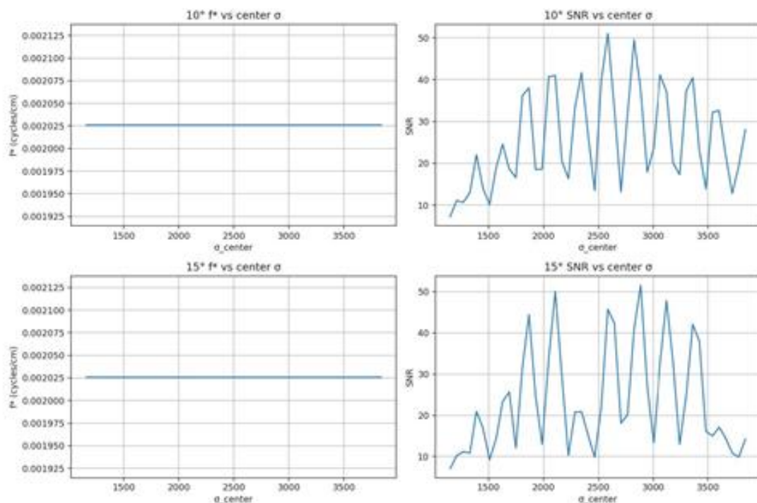
图5 全带滑窗 FFT 结果图
