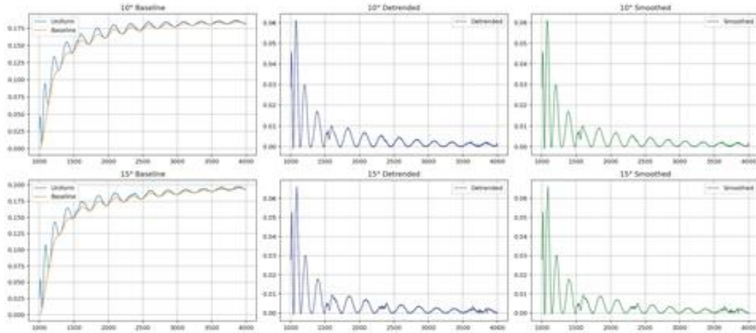
图 4 去趋势化、去噪后数据图
