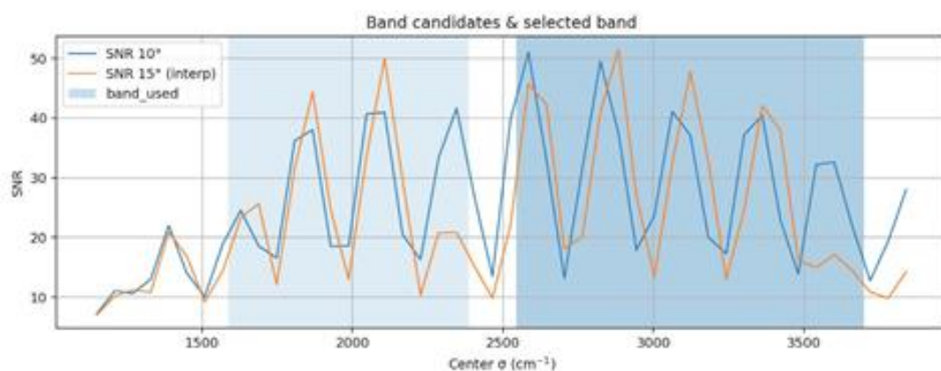
图6 有效频段选择
