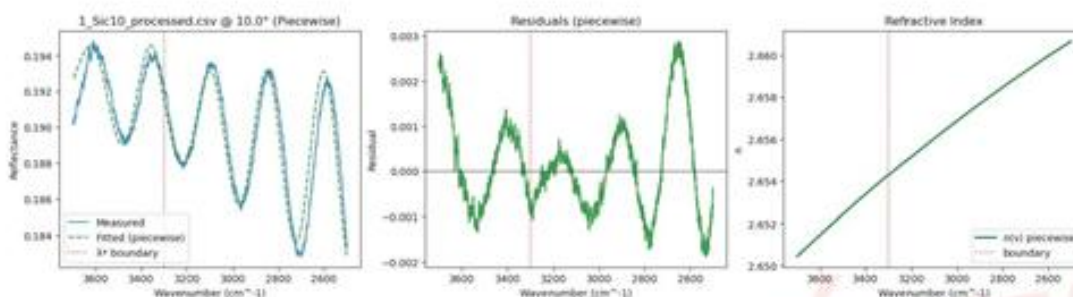
图 10 10 度-SiC 分段拟合结果
