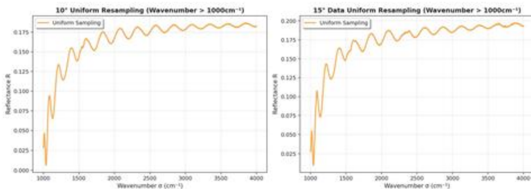
图3 裁剪低波数区域后等间距重采样图
