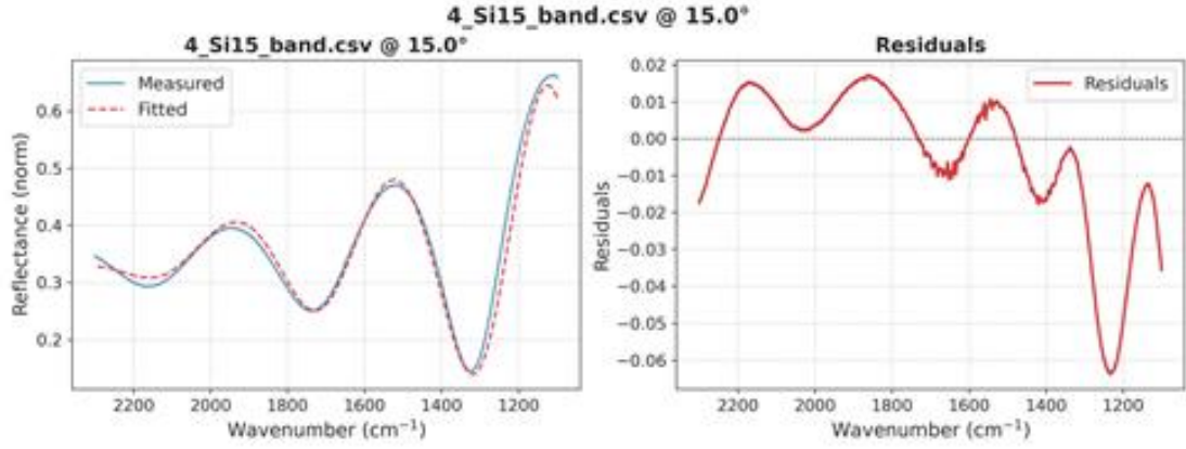
图 31 15 度-Si 拟合结果
