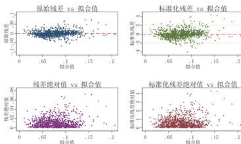
图 10 同方差性检验
