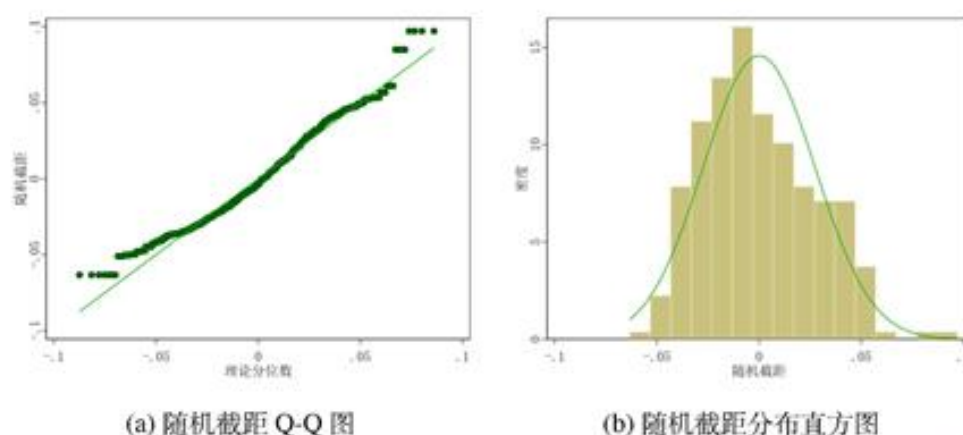
图 9 随机截距正态性检验
