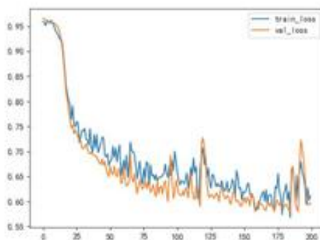
图 17 模型训练损失
