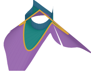
(d) Reflected annuli and closure
